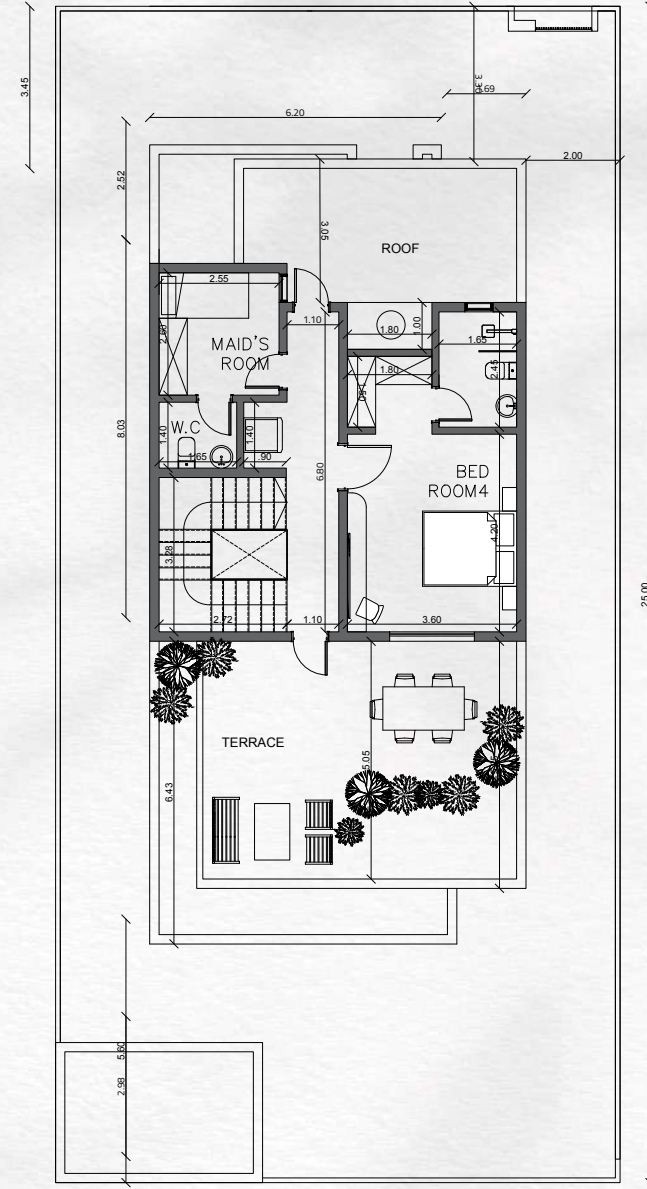
الدور العلوي ROOF FLOOR
