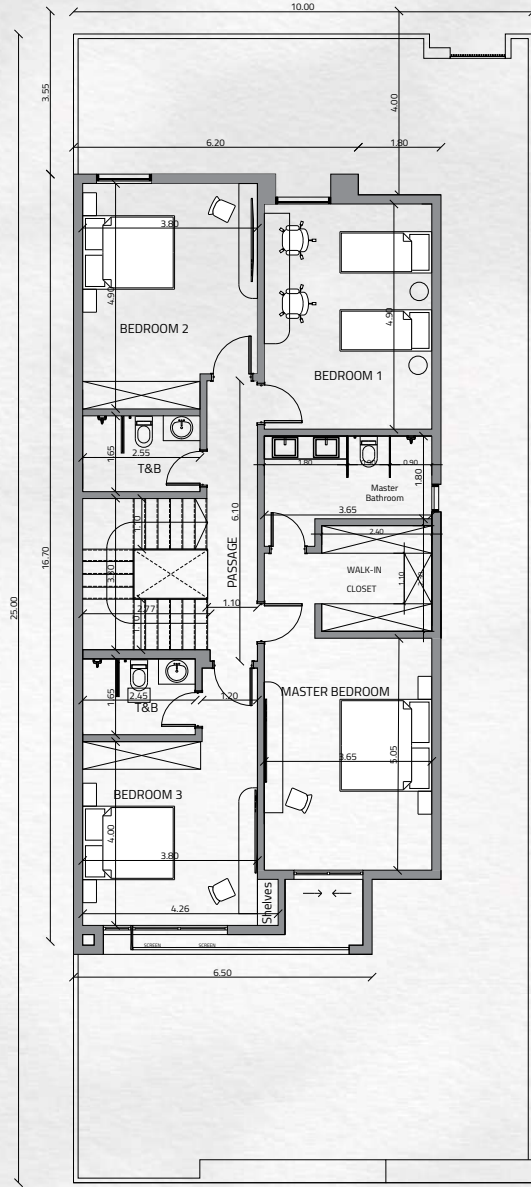
الدور الأول FIRST FLOOR
