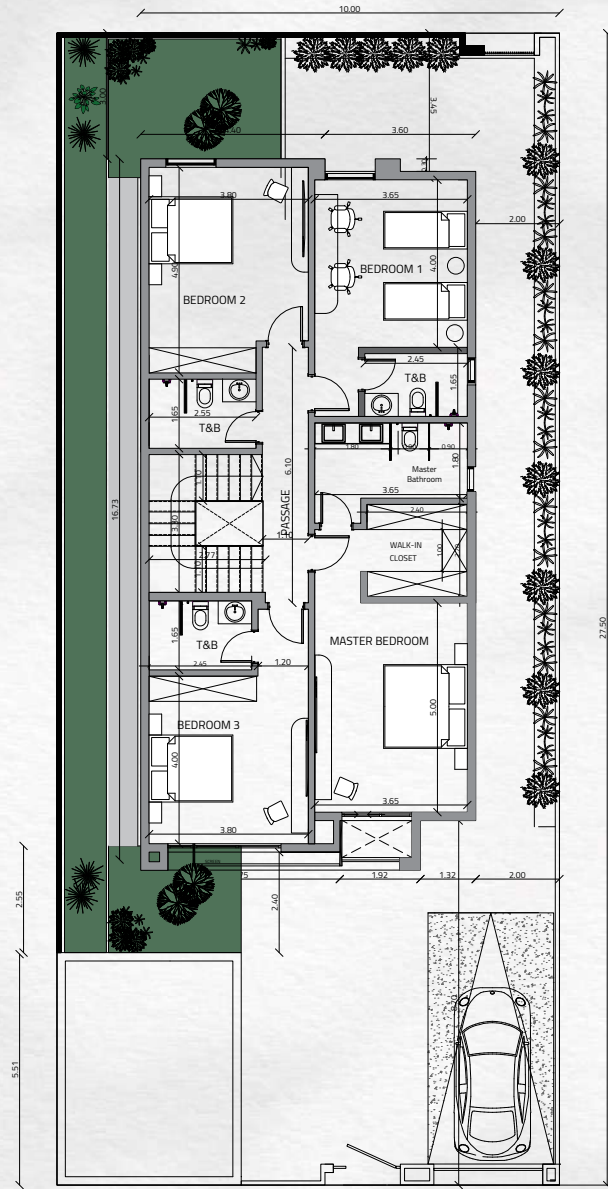
الدور الأول FIRST FLOOR
