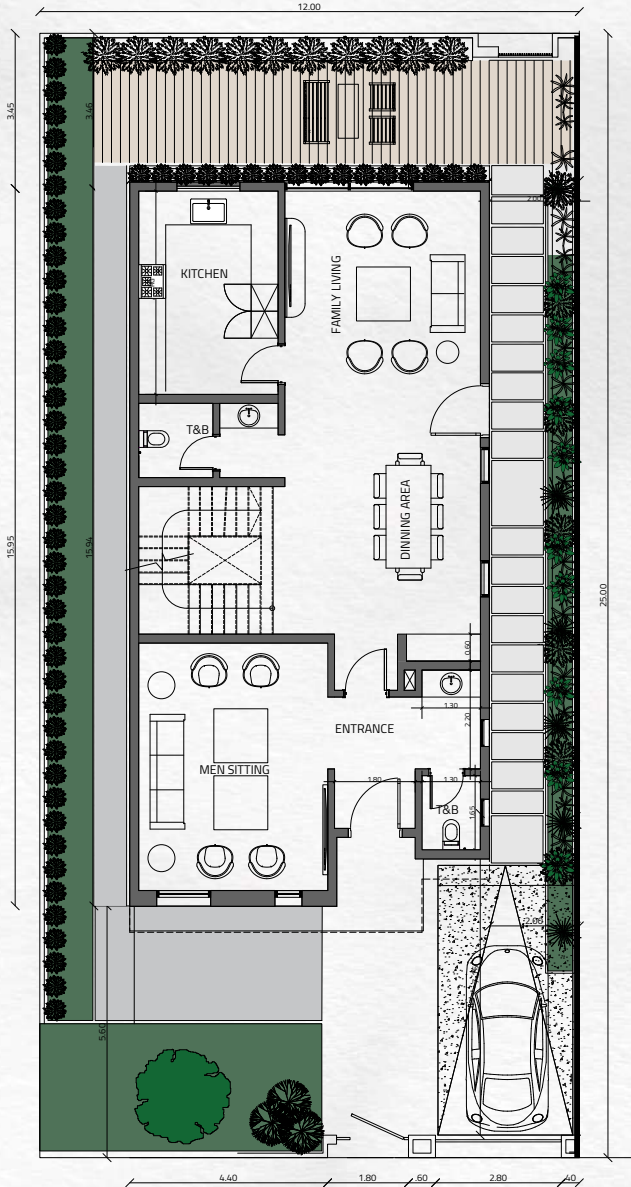
الدور الأرضي GROUND FLOOR
