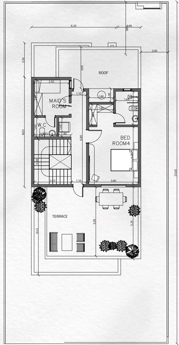
الدور العلوي ROOF FLOOR
